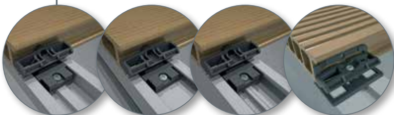
Montáž pomocí spon
